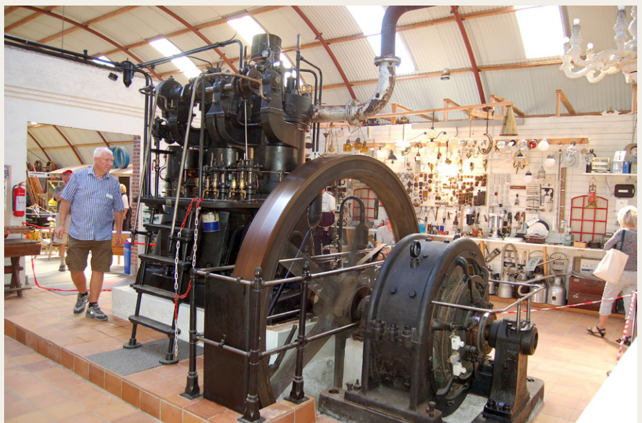
På Bornholms Tekniske Samling så vi blandt andet dette gamle elværk fra Poulsker. det drives af en to-cylindret firtakts B&W dieselmotor. Dynamoer kommer fra Thrige i Odense.
