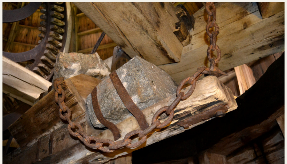
Datidens „elektronik“ i form af nobremse til vingerne.
