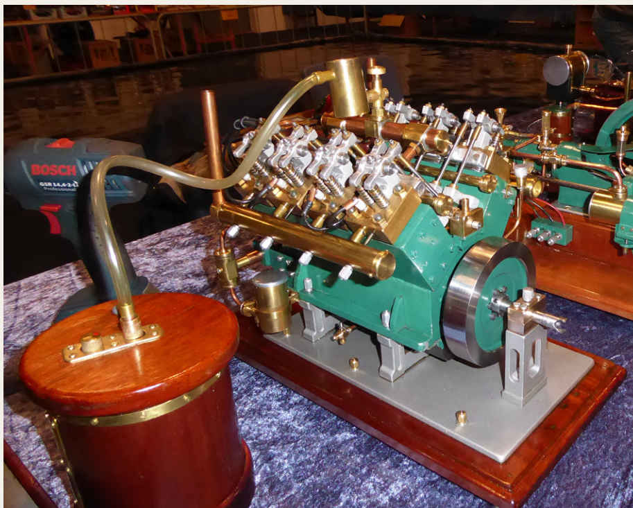
En meget fin og velfungerende V8 motor fremstillet af Henry Nielsen fra Thy.
