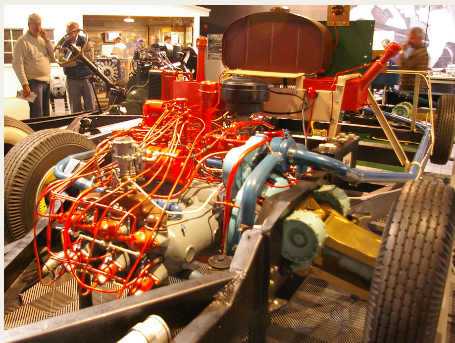
Den store 9,7 liter eksperimentalmotor med de hydraulisk aktiverede ventiler, der afstedkom en rørføring, man med rette kan benævne „fuglerede“. Det høje arbejdsstryk, der var krævet af hydraulikken, fordrede et 24V spændingsystem, og i tilgift skulle motoren køres alt for længe på starteren, før arbejdsstrykket var tilstrækkeligt højt til, at motoren kunne starte.
