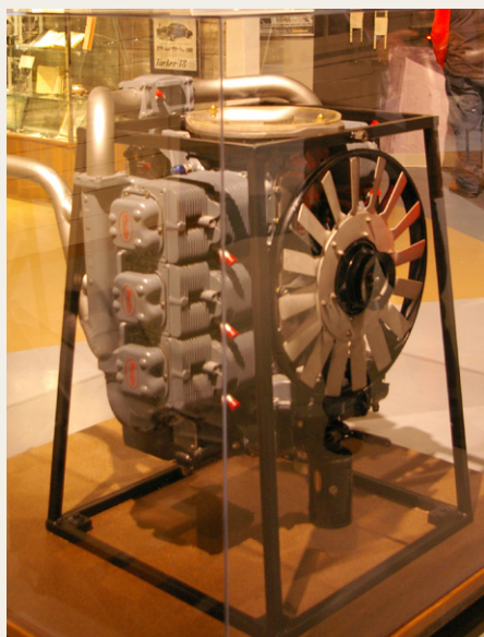
Franklin helikoptermotoren som i kraftig modificeret form blev anvendt til Tucker '48.
