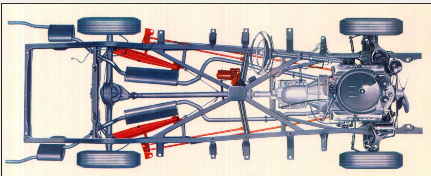
På denne illustration fra brochuren er affjedringssystemet vist i rødt. Vi ser de lange torsionsstænger, som forbinder forhjulspængene med baghjulspængene. Midt under bilen sidder motoren, som regulerer højden på bilens bagende.
