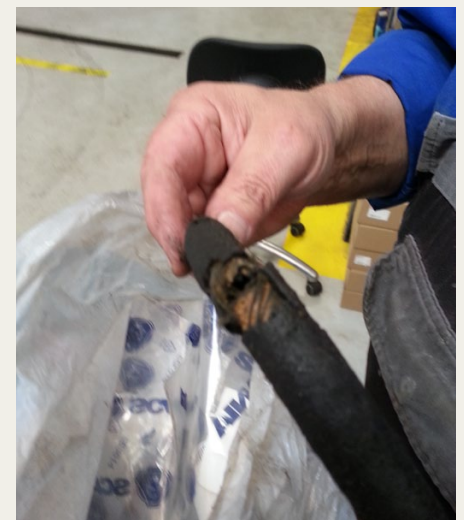
En af de slanger som leverede luft til gearkasse og døre.
